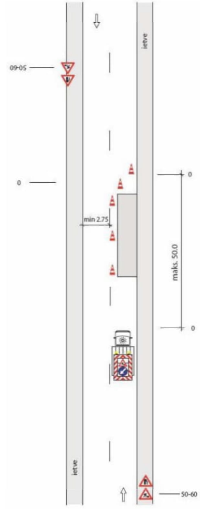
12. SHĒMA Islaicīgo darbu vieta, norobežota ar pārvietojamo ceļa zīmju vairogu.
